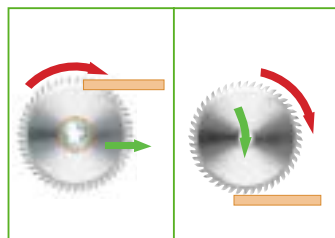
Optimale, gelijkmatige ingrijphoek. Ongunstige hoek bij het invallen.
