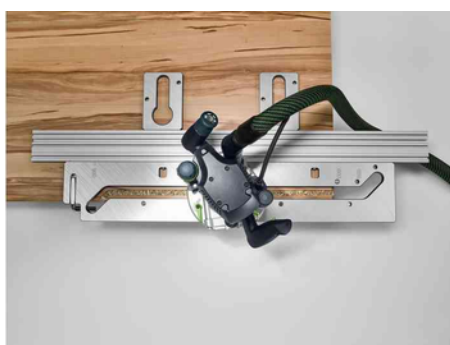
Werkplaatssjabloon APS 900/2 voor hoek- en platenverbindingen tot 900 mm diepte 204219
