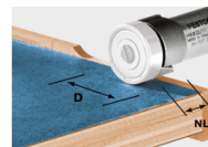
Aanloopkogellager KLS- D 15,8 -OFK voor frees 490090, 490091, 490092, 490093, 490094, 490095, 490096, 491533 Bestelnummer 490249
